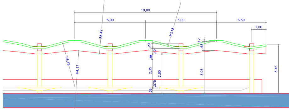
VISTA FRONTAL ESC: 1:50
