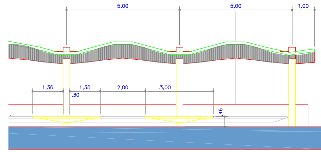
VISTA FRONTAL ESC: 1:50
