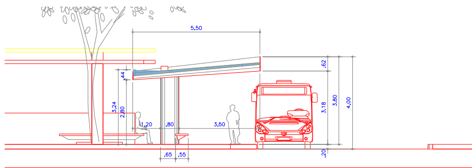
SECCION LATERAL ESC: 1:50
